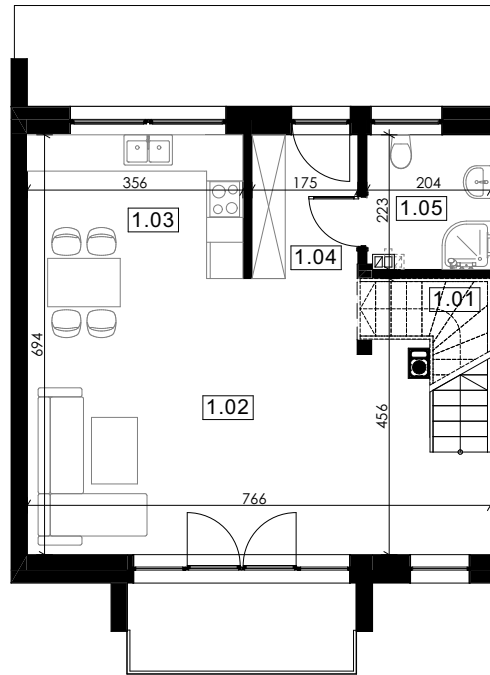
KONDYGNACJA 0
